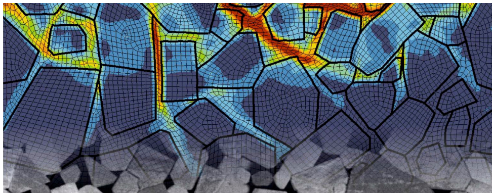
Simulation de champ de pression sur granulat polycristallin appliquée à un problème de tribologie.
