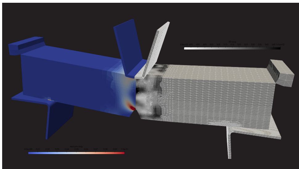
Théorie et pratique : confrontation entre simulation numérique et essai mécanique en comportement fortement non-linéaire.
