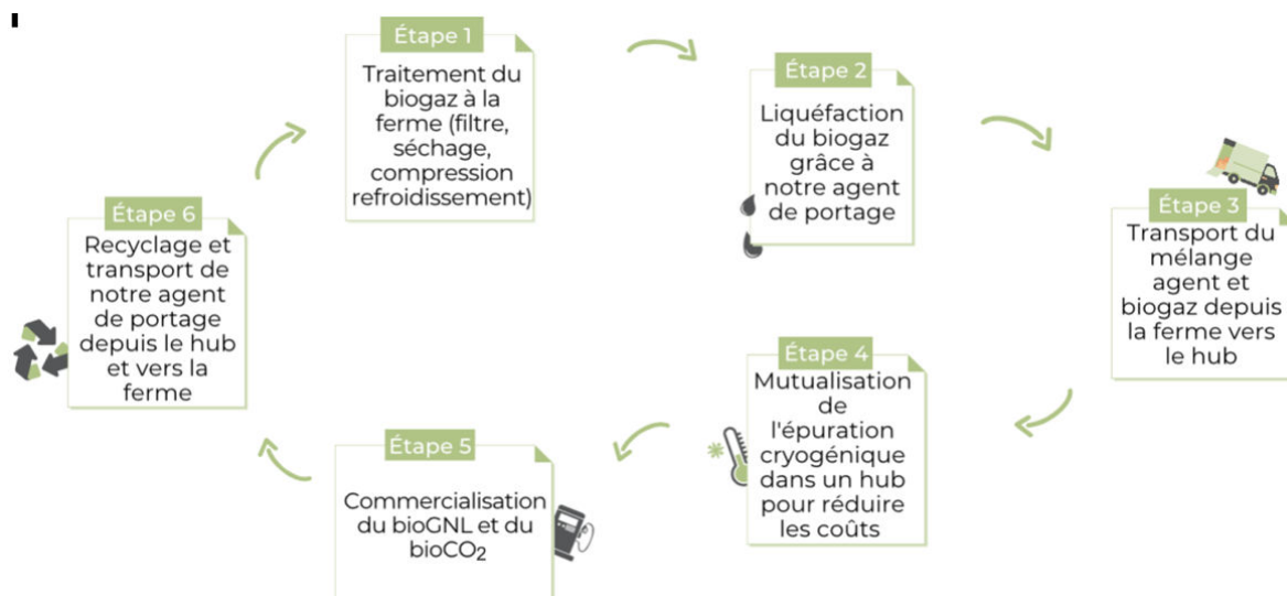
Schéma illustrant le processus technique de SUBLIME Energie
